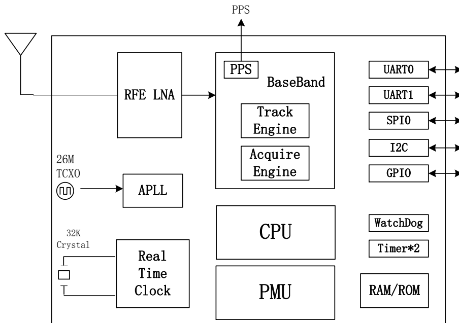
图 1-2 模块框图
