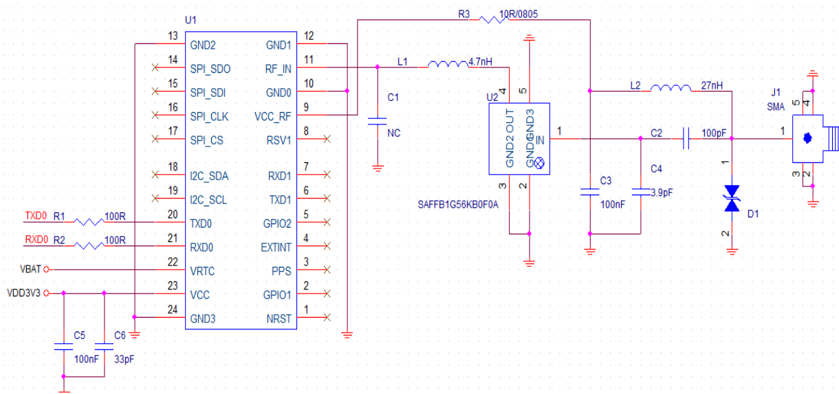
图 7-2 MXT901E 模块内部馈电参考设计
