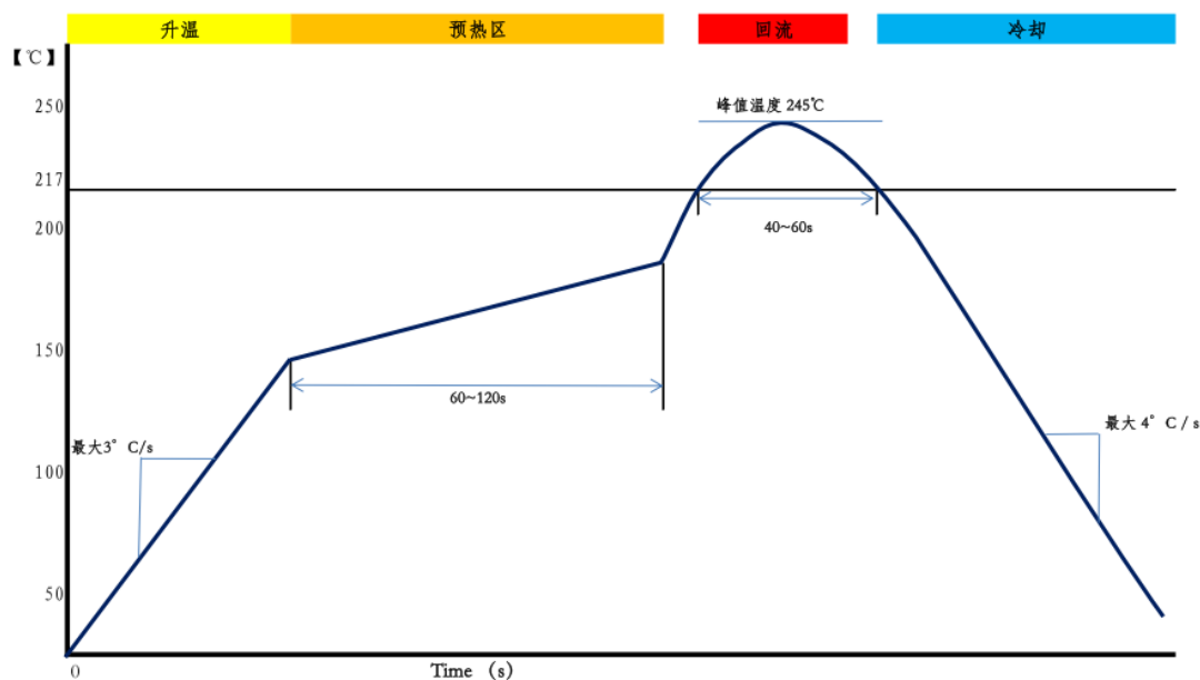
图 8-1 MXT901E 推荐炉温曲线
