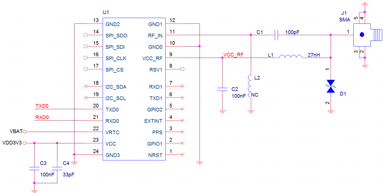
图 7-1 MXT901E 参考设计
