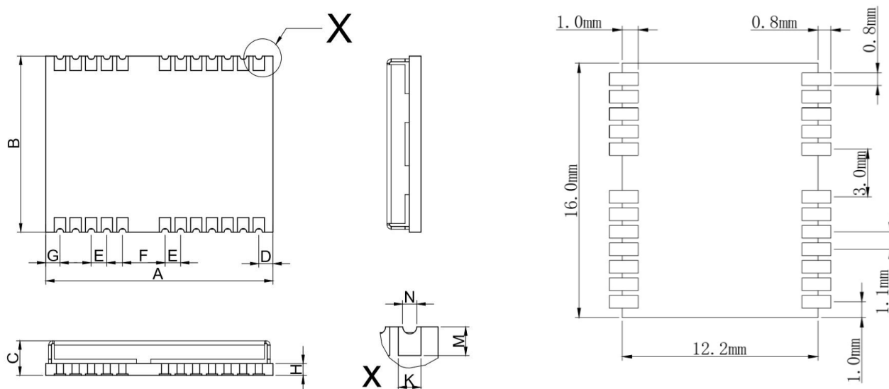
图 6-1 MXT901E 外形尺寸及 PCB 封装参考
